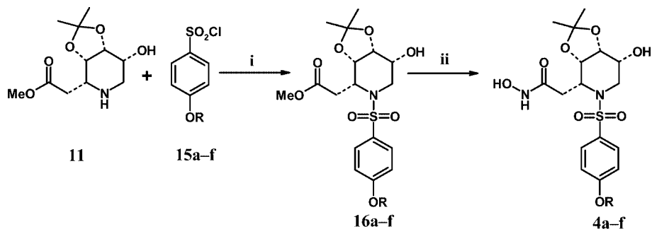
Scheme 3. (i) \text{K}_2\text{CO}_3 , \text{CH}_3\text{CN} ; (ii) \text{NH}_2\text{OK} , \text{CH}_3\text{OH} .
